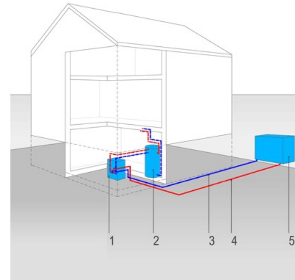
1: Wärmepumpe Inneneinheit 2: Pufferspeicher 3: Rücklauf 4: Vorlauf 5: Außengerät mit Ventilator und Verdichter
