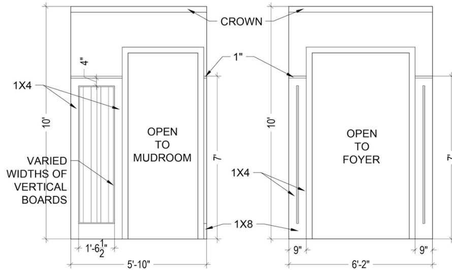
A HALLWAY ELEVATION SCALE: 3/8" = 1'-0"
