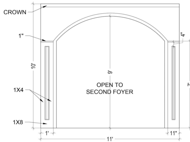
C Foyer Elevation SCALE: 3/8" = 1'-0"
