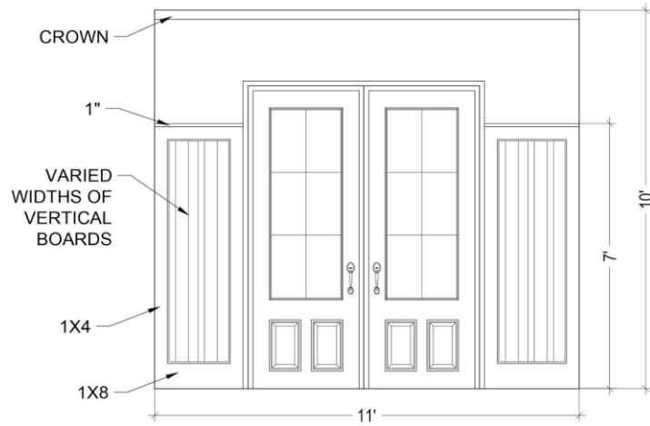
A Foyer Elevation SCALE: 3/8" = 1'-0"
