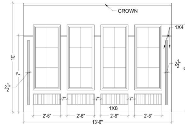
E DINING ROOM ELEVATION SCALE: 3/8" = 1'-0"
