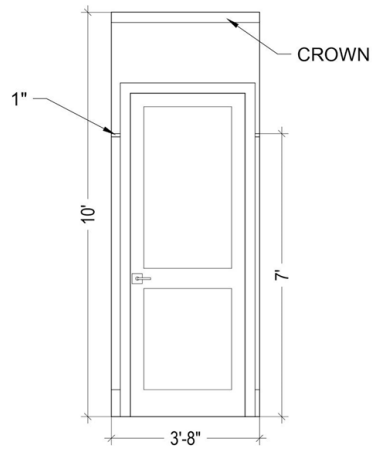
MUDROOM ELEVATION SCALE: 3/8" = 1'-0"
