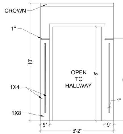
D Foyer Elevation SCALE: 3/8" = 1'-0"
