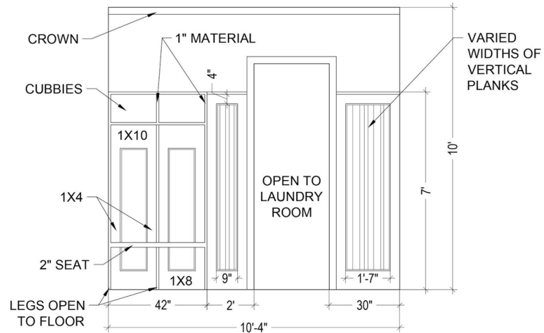
MUDROOM ELEVATION SCALE: 3/8" = 1'-0"
