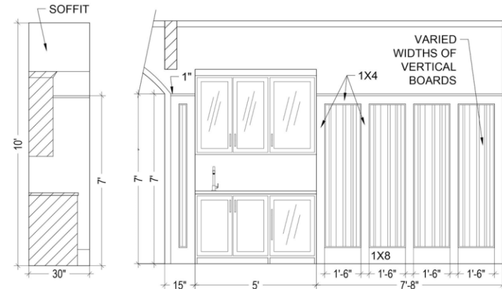
C DINING ELEVATION SCALE: 3/8" = 1'-0"
