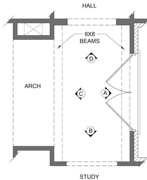
FOYER - FLOOR PLAN SCALE: 3/8" = 1'-0"
