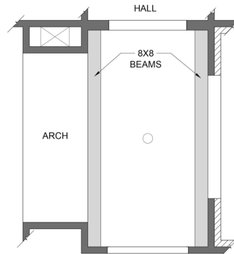
FOYER - RCP SCALE: 3/8" = 1'-0"
