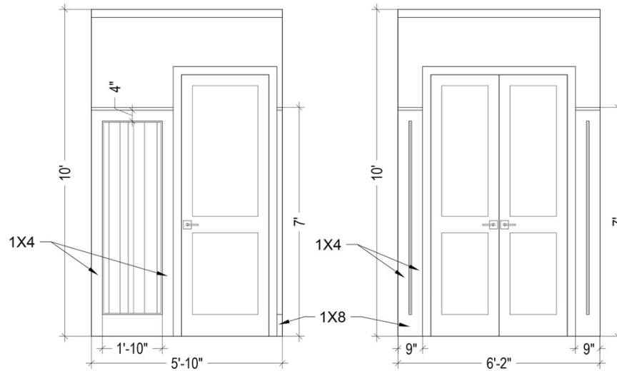
C HALLWAY ELEVATION SCALE: 3/8" = 1'-0"
