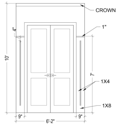
B Foyer Elevation SCALE: 3/8" = 1'-0"
