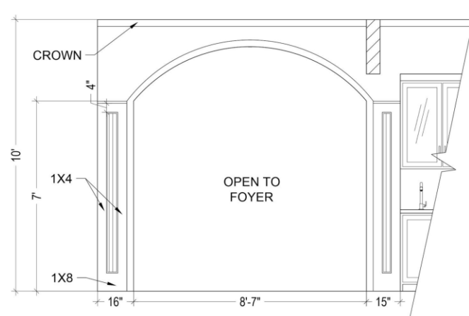
E SECOND FOYER ELEVATION SCALE: 3/8" = 1'-0"
