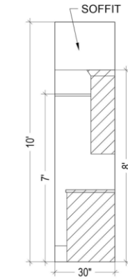
B DINING ELEVATION SCALE: 3/8" = 1'-0"
