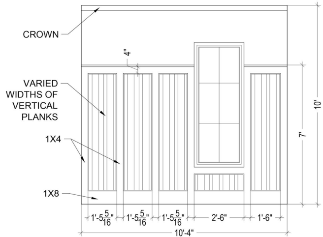
MUDROOM ELEVATION SCALE: 3/8" = 1'-0"
