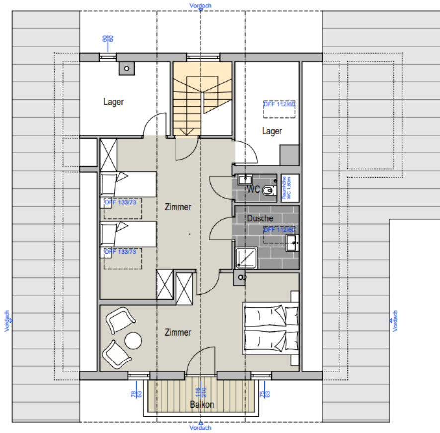
3e Obergeschoss
