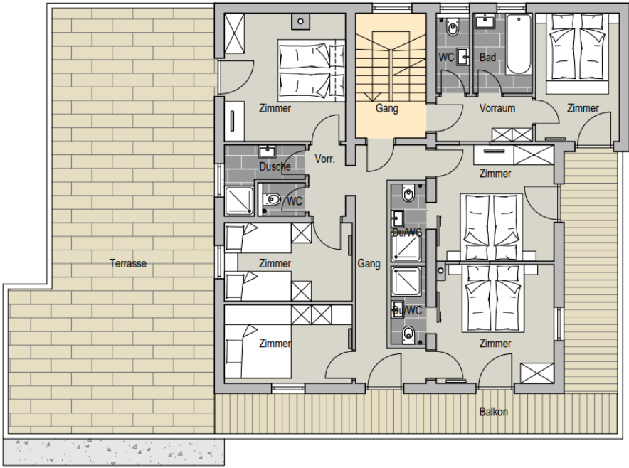
1e Obergeschoss
